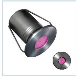
HLO-6202 (3W) - RGB Size : Ø68.5x73mm
