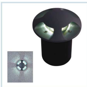
HLO-6854 (3W) Size : Ø120x150mm
